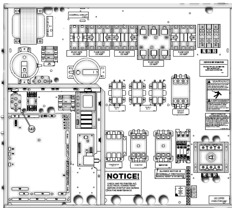
EP FAN COIL FUSED
