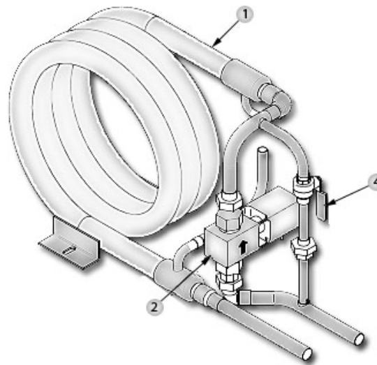
3 TON 2 WAY HP
